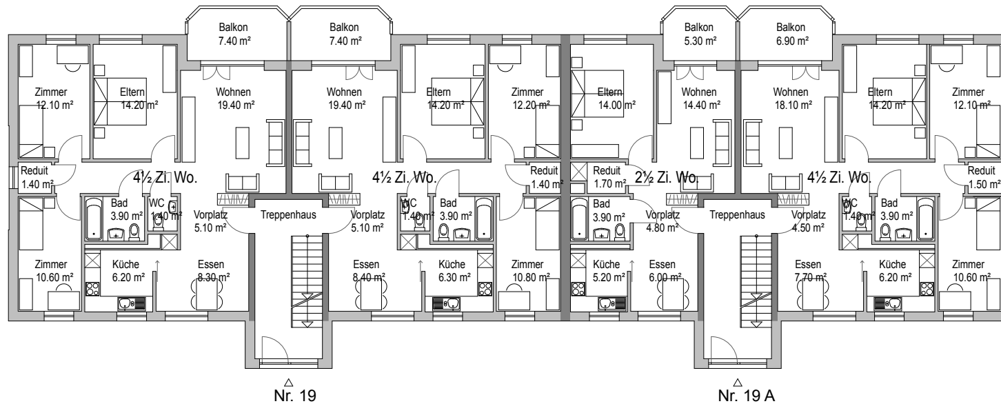
Steinackerweg 19 / 19 A Grundriss Erdgeschoss
