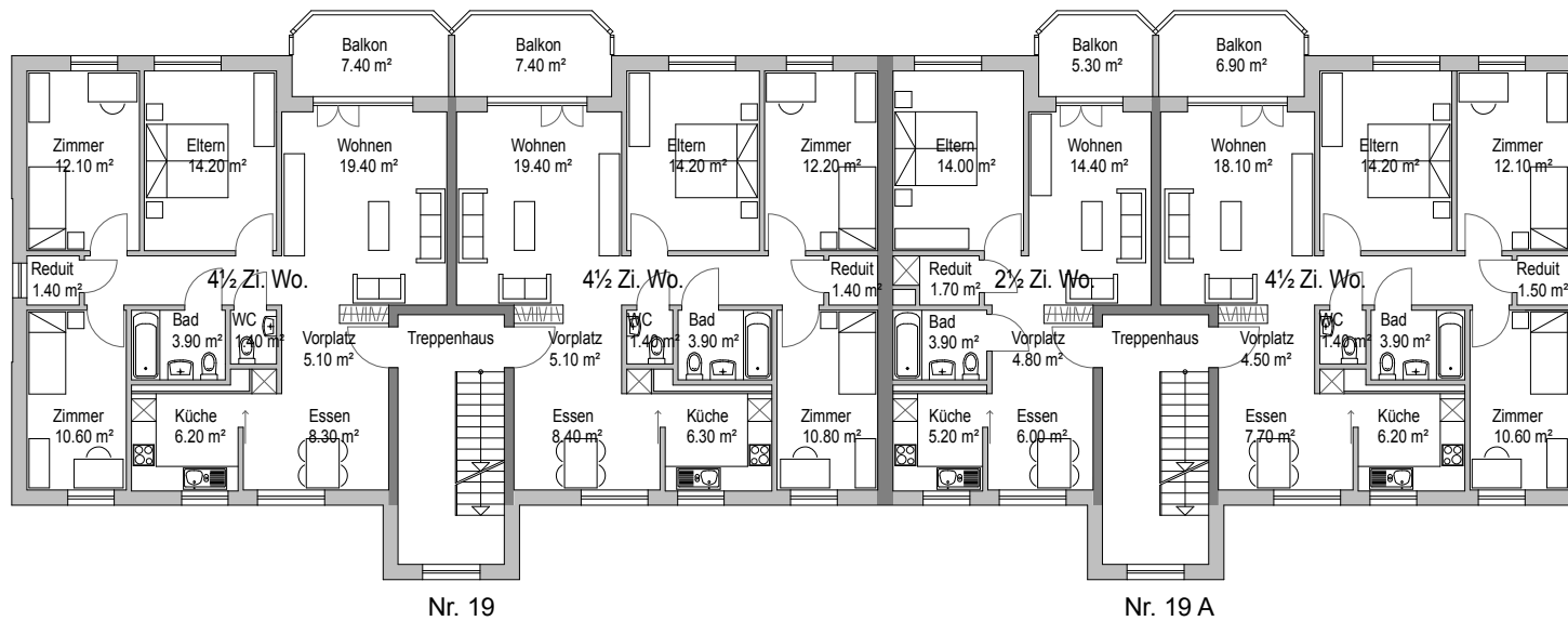
Steinackerweg 19 / 19 A Grundriss 2. Obergeschoss
