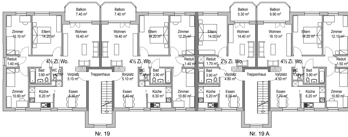
Steinackerweg 19 / 19 A Grundriss 1. Obergeschoss
